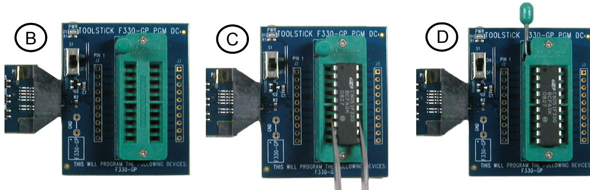
Figure 10. ZIF Socket
